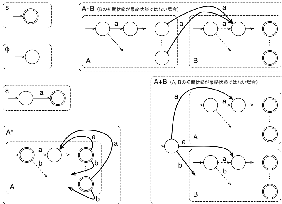
図 3.7 正規表現から有限オートマトンへの変換
