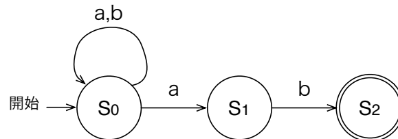
図 3.5 非決定性有限オートマトンの例
